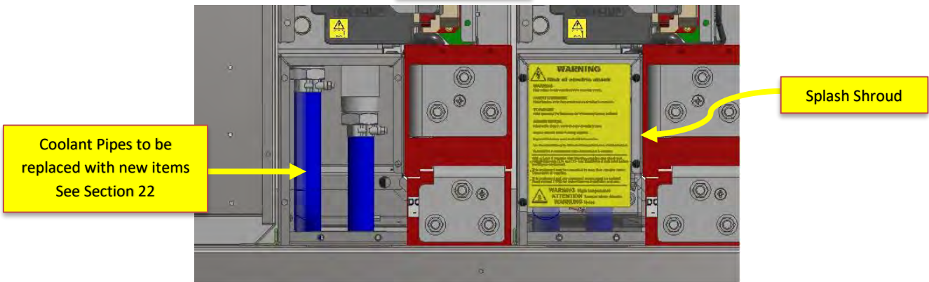
GEN CABINET
