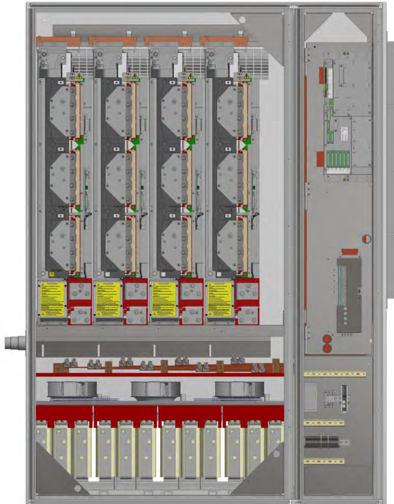
GEN CABINET
